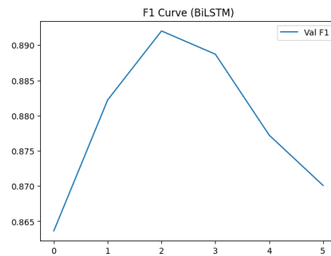
(B) BiLSTM
